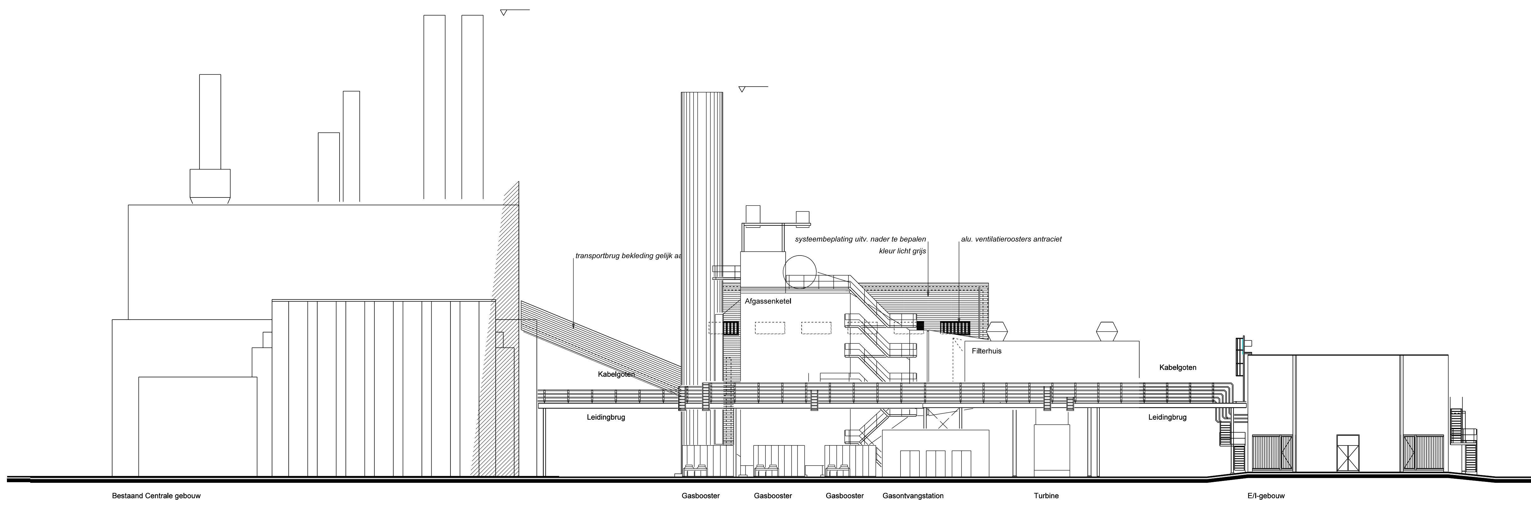
aanzicht westzijde
